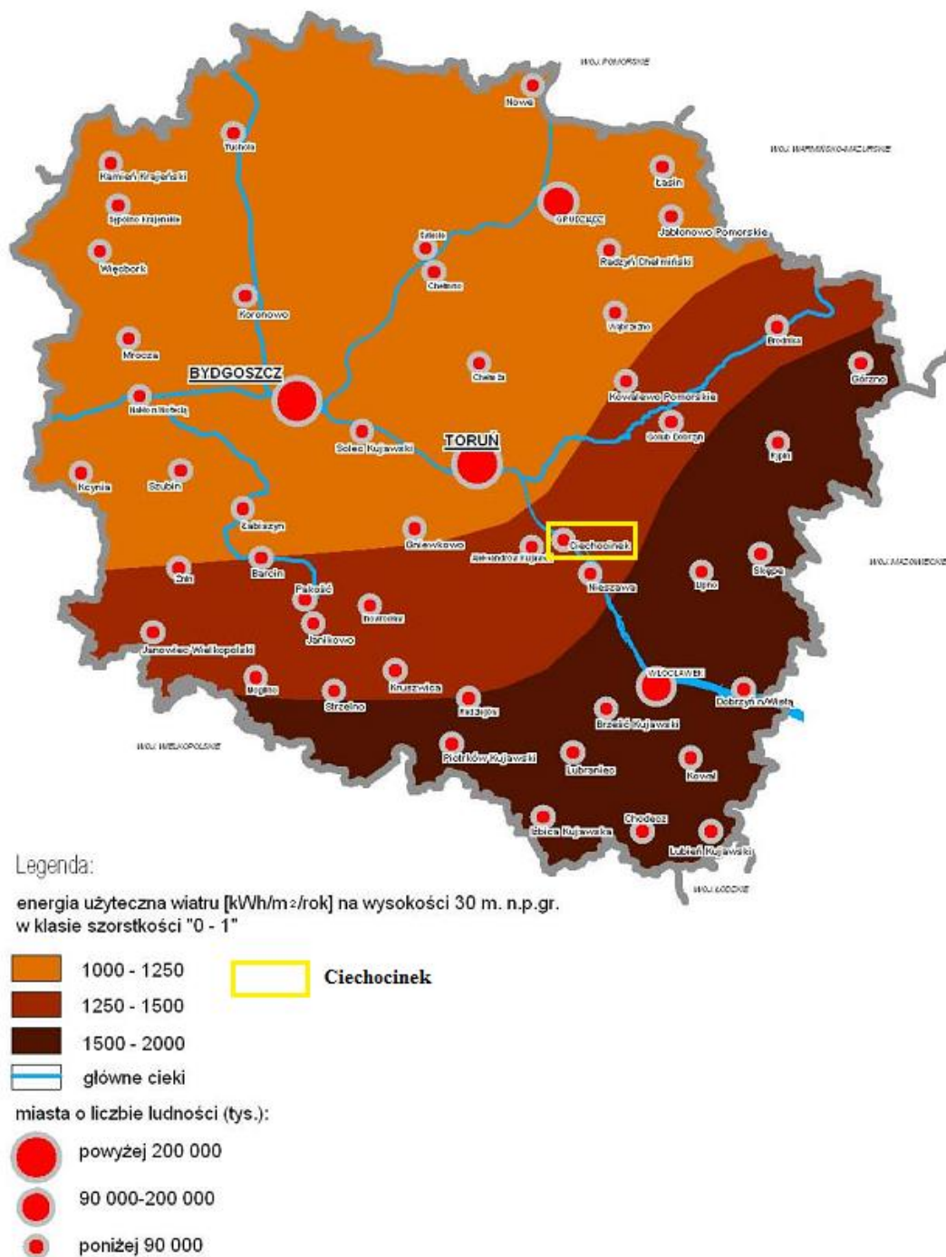
Rysunek 8. Strefy energetyczne wiatru - energia użyteczna wiatru w województwie kujawsko - pomorskim.
